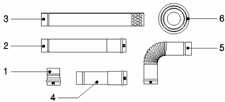
Εξαρτήματα καμινάδας
